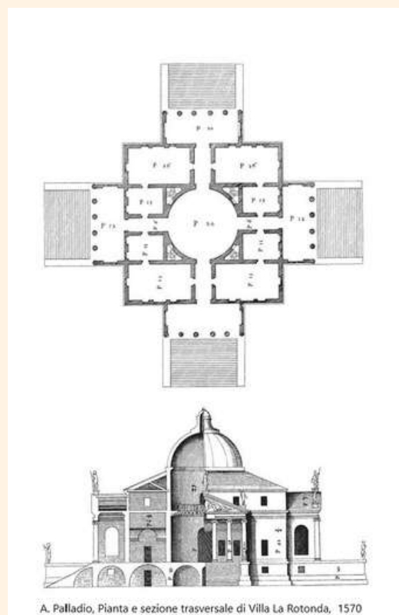
A. Palladio, Pianta e sezione trasversale di Villa La Rotonda, 1570
